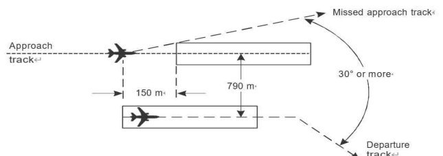
그림 6-9. 도착 항공기로부터 멀어지도록 활주로의 이격된 경우의 분리평행운영 (6.7.3.6.2 참조)
