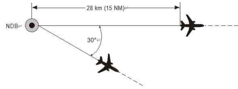
그림 5-5. 동일 무지향표지시설(NDB)을 이용한 분리 (5.4.1.2.1.2 나) 참조)
