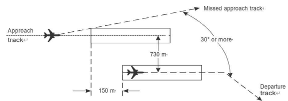
그림 6-8. 활주로의 도착 항공기를 향해 이격된 분리평행운영 (6.7.3.6.2 참조)
