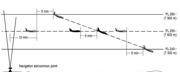
그림 5-18A. 상승하는 항공기와 동일 진로 상 항공기 간 5분 분리 (5.4.2.2.2.1 다) 2) 참조)
