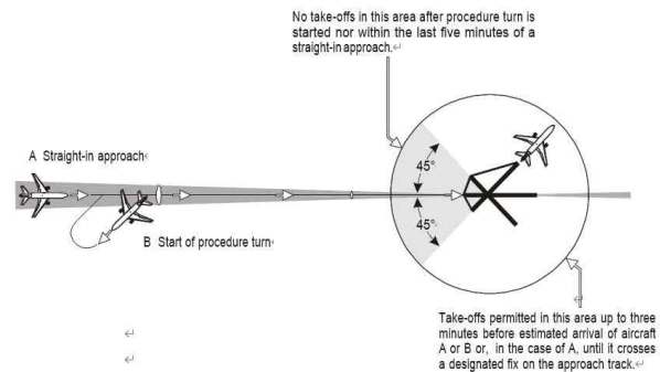
그림 5-41. 도착 보호구역의 예시
