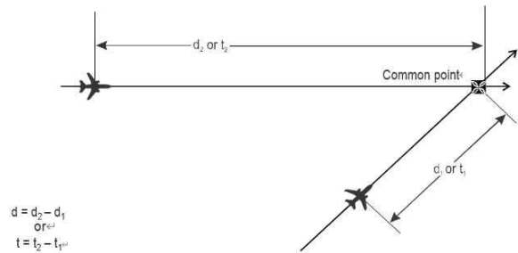
그림 5-32. 동일진로이나 일치하지 않는 항공기 간 종적인 거리/시간의 계산
